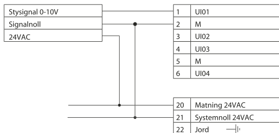
Inkopplingsexempel Inkopplingsexempel för aktiva givare på ingångarna UI01 - UI04
