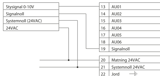
Inkopplingsexempel Inkopplingsexempel för ventilmotorer
